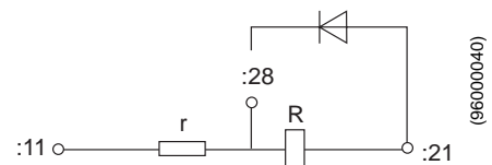
Fig. 2 RXMS 1
